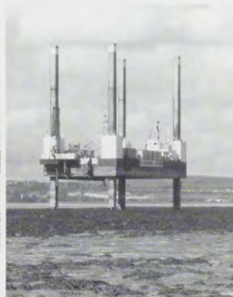
Grondonderzoek
