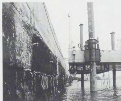
Grout injecties
